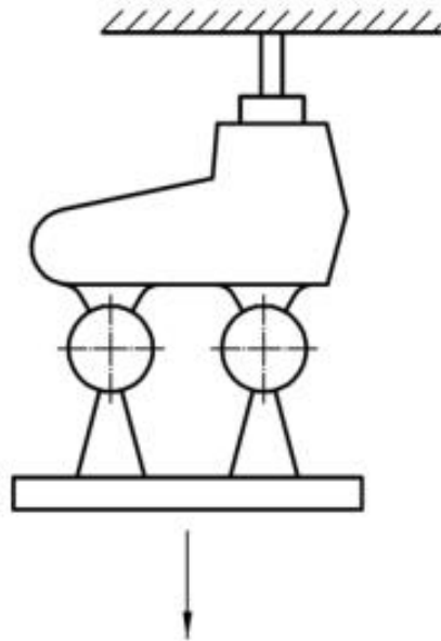
그림 3 - 신발이 연결된 차대의 부착 강도(인장 힘 방향)
